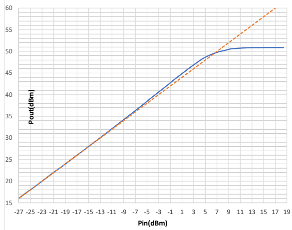
P1dB
