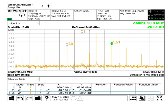
2 tones 47dBm ave / 50dBm peak at 960MHz
