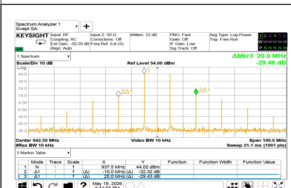
2 tones 47dBm ave / 50dBm peak at 942.5MHz
